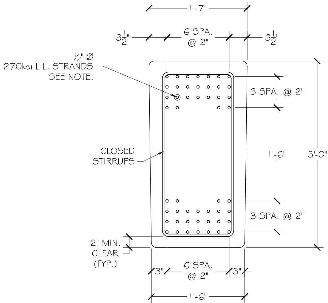
TYP SECT 18" x 36" BEAM CROSS SECTION SCALE: N.T.S.
